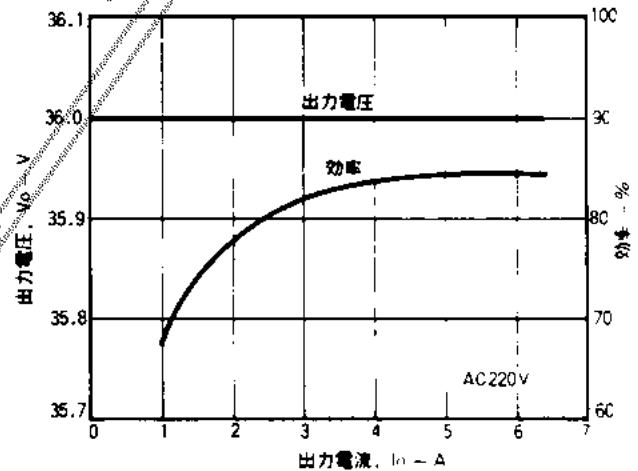
出力電圧, 効率 - 出力電流
