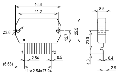
外形図 4199
