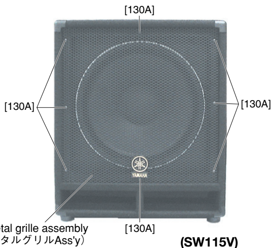
[130]: TH Sheet Metal Screw (トラスタップねじ) #6 x 5/8 BLK (WJ493800)
